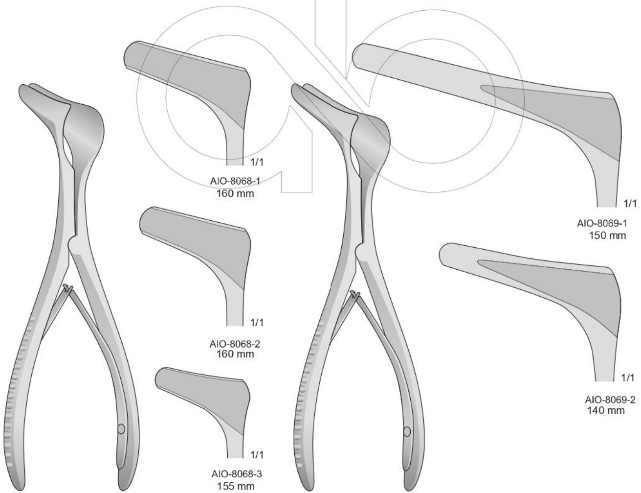
HARTMANN AIO-8068
