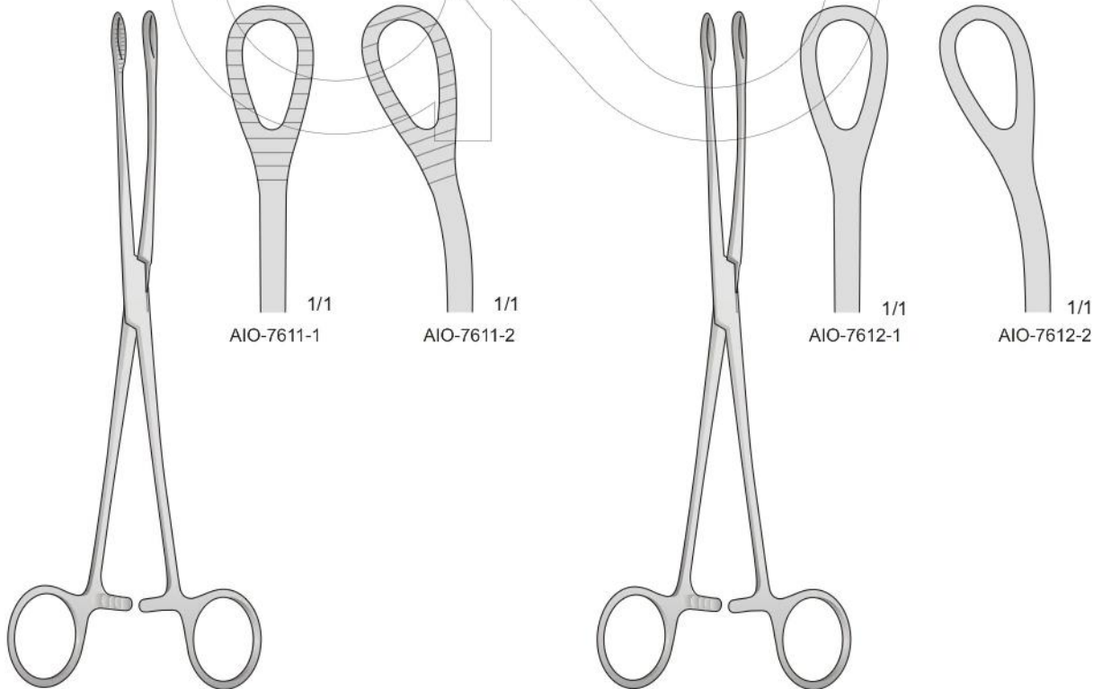
FOERSTER-BALLENGER AIO-7611 240 mm
